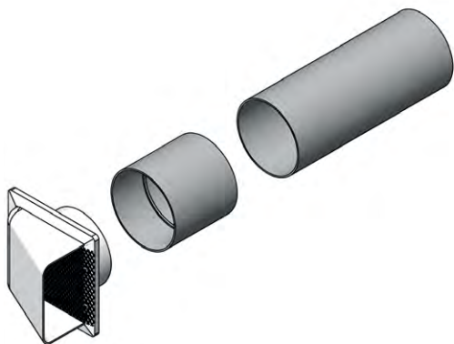
Paloilmaliitännä standard: sokkelin/seinän läpivientisarja IA-AIR00-000 putki Ø 100mm, pit. 250mm kaulus pit. 100mm
