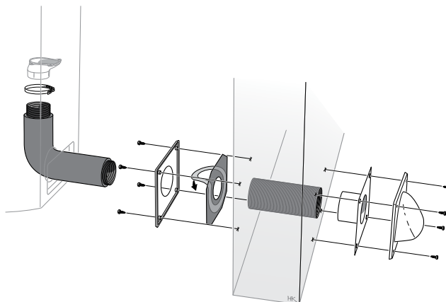
Paloilmaliitännä: sokkelin/seinän läpivientisarja, kondenssieriste & putki IA-80655-200
